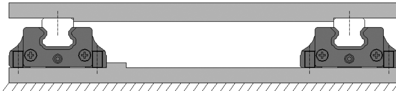
(B) Auf horizontaler Ebene mit festen Gleitstücken (B) На горизонтальной поверхности с закрепленными блоками
